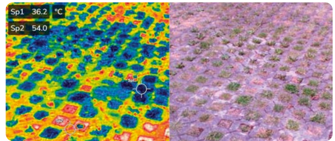
Begrüntes Rasengitter als Parkplatz (Vegetationsbereich mit 36,2°C und Betongitter mit 54°C)
