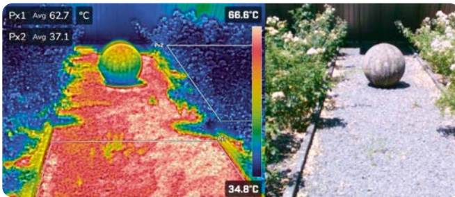
Schottergarten mit angrenzendem Rosengarten (Schottergarten mit 62,7°C und Rosengarten mit 37,1°C)
